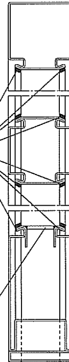
Schnitt 1 - 1
