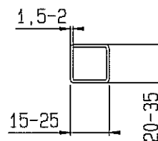
Glashalteleiste Vk-Rohr
