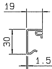
Glashalteleiste 19mm Art.170032
