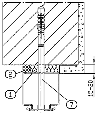
Durchsteckdübelmontage
