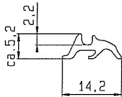
Dichtkeil 3 mm Art.-Nr. 179005-1
