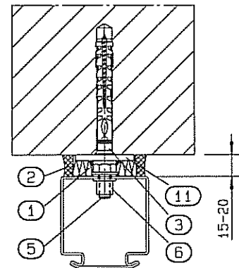
Anschweißmontage Porenbeton
