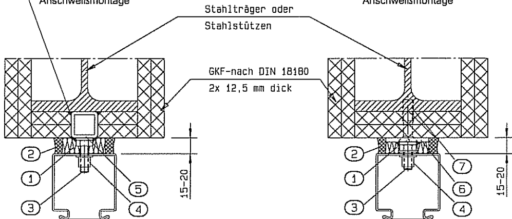
Anschweißmontage
