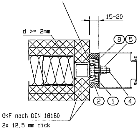
Anschweißmontage seitlich
