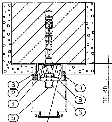
vormontiertes Einputzanschlussprofil
