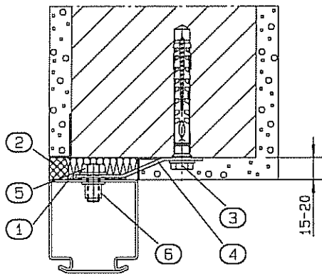
Ankermontage mit Dübellasche
