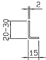
Winkelglashalteleiste Art. 170049
