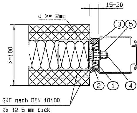
Anschweißmontage seitlich
