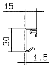
Glashalteleiste 15mm Art.170002
