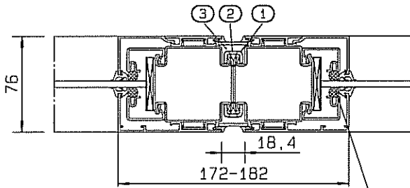
Ausführung A (Stahl/Alu)
