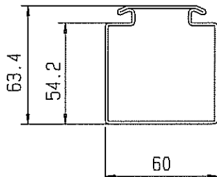
Rahmenprofil Art.270007
