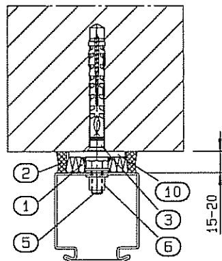
Anschweißmontage Sichtmauerwerk
