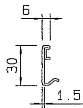
Glashalteleiste 6mm Art.170031a
