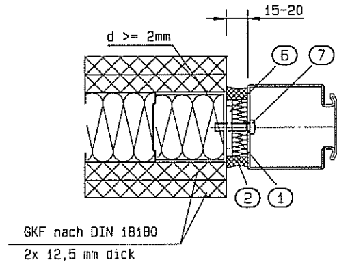
Anschweißmontage seitlich
