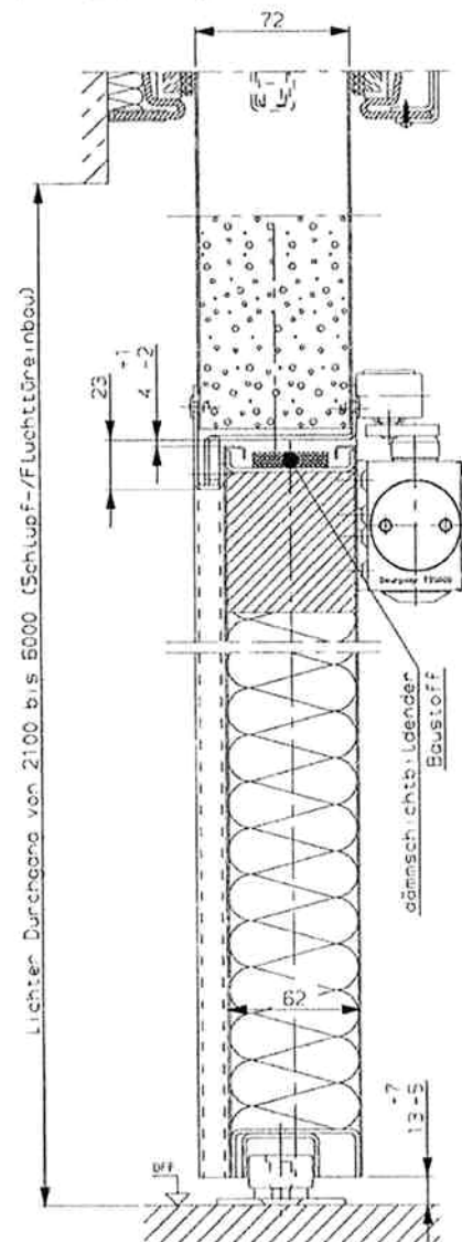
Schnitt B-B
