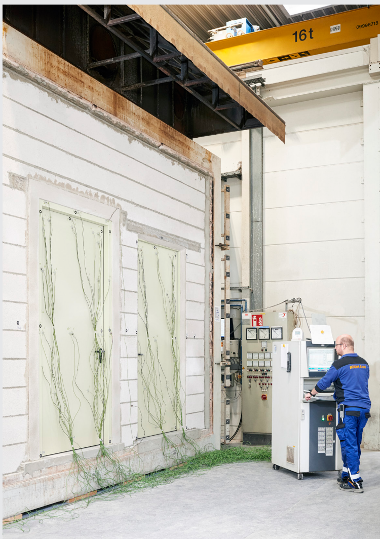
Brandschutztest der Türen im Prüflabor des hauseigenen Brandschutzzentrums
